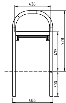
DRAHTGITTER
